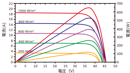
RSM132-8-665M 異なる照射量下での I-V カーブ
