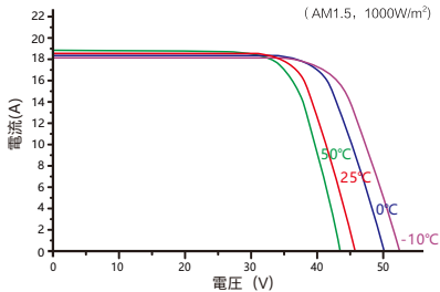
異なる温度下での I-V カーブ (AM1.5, 1000W/m²)
