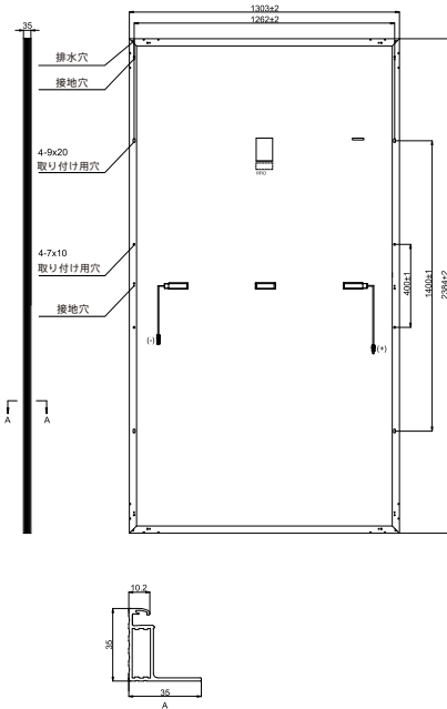
太陽光発電モジュール図面 単位:mm
